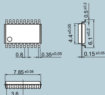
SSOP-20
