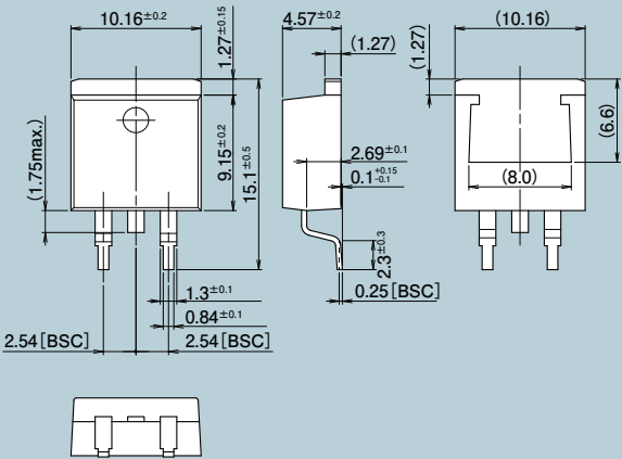
D2-Pack
